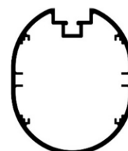
Alu-Profil 120 x 100
