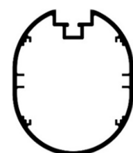
Alu-Profil 120 x 100
