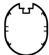
Alu-Profil 120 x 100
